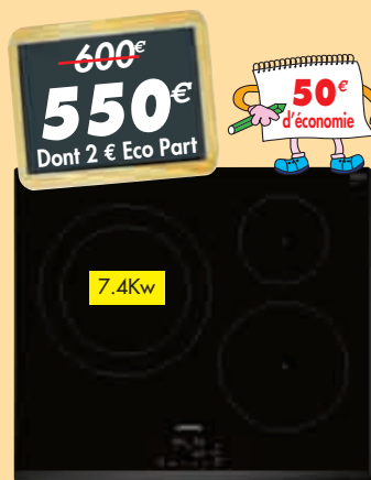
SIEMENS EH 651BJB1E TABLE DE CUISSON 3 inductions dont 1 double zone 28 cm avec Boosters, 3 Timers, commandes TouchControl.
